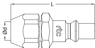
Plug / Nippel
