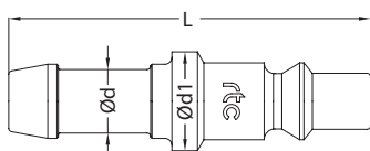
Plug / Nippel
