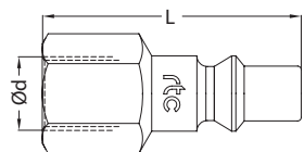
Plug / Nippel
