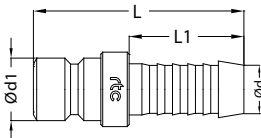
Plugs / Nippel
