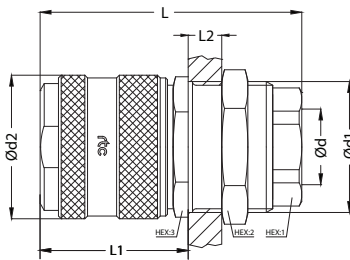
Socket
