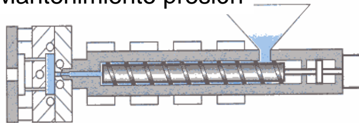
Mantenimiento presión
