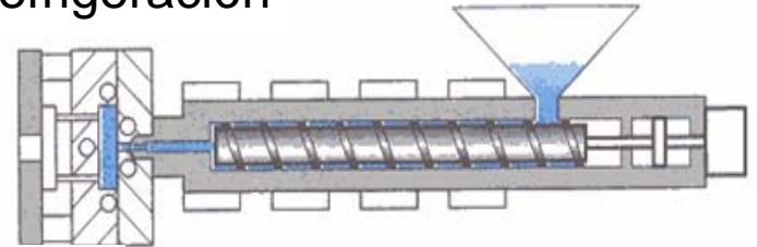
Refrigeración
