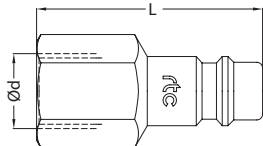
Plug / Nippel
