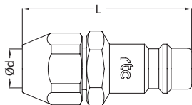
Plug / Nippel
