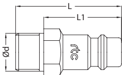
Plug / Nippel
